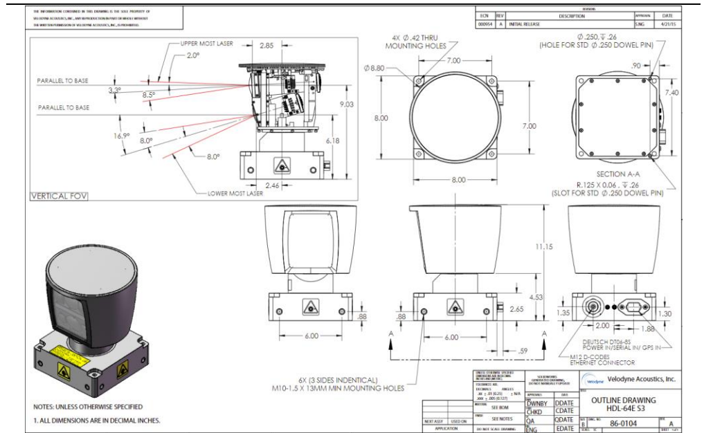
图 10 Velodyne 64 线激光雷达结构
