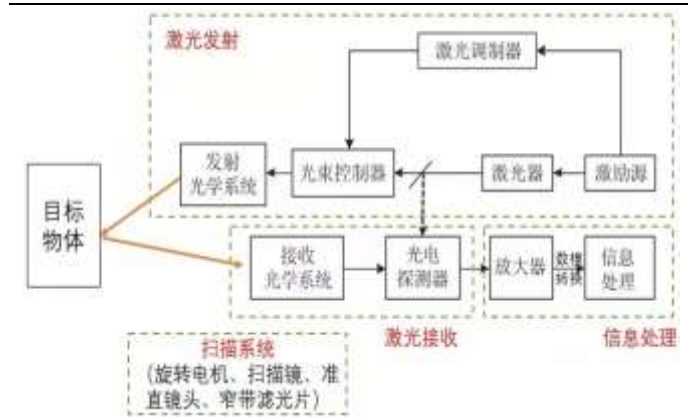
图 7：激光雷达的工作原理
