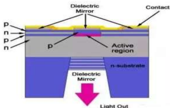
图 11: 垂直腔面发射激光器 (VCSEL) 结构图
