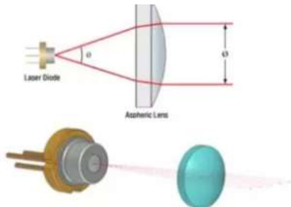
图 12: 透镜系统结构图
