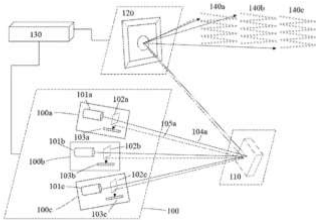
图 17: 华为激光雷达的光路图
