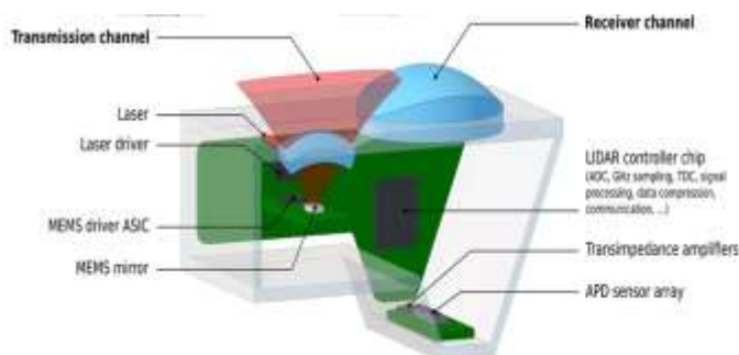
图 15: MEMS 激光雷达结构
