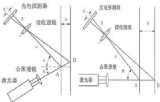
图 10：三角式激光雷达测距原理
