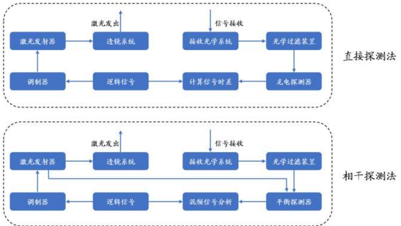
图 13: 直接探测法与相干探测法的基本原理
