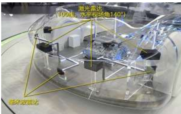
图 5：华为于上海车展中展示的激光雷达方案
