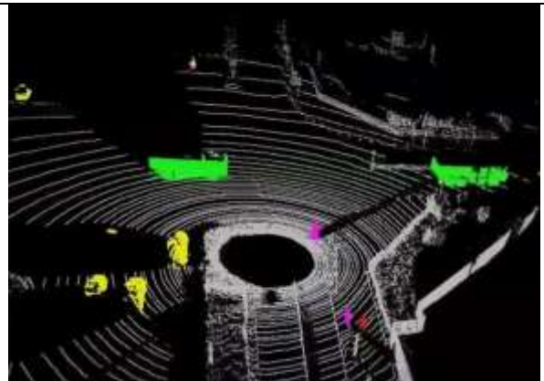
图 8：激光雷达在街道环境生成的点云数据渲染图
