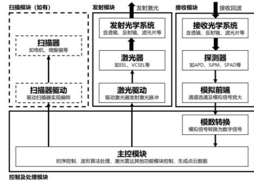
图 2 ToF 激光雷达核心模块示意图
