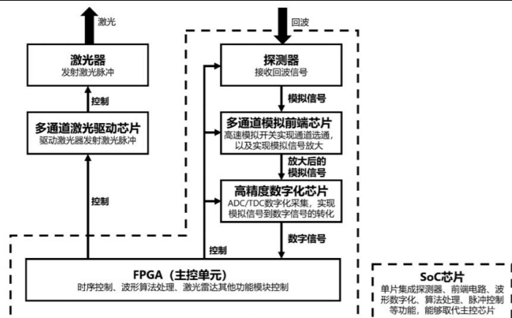
图 10 激光雷达专用芯片及功能模块示意图
